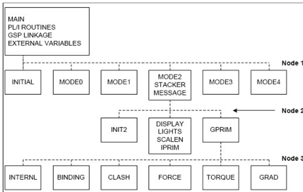
Рис. 15.1 Граф структуры программы (пример W. V. Wright)
