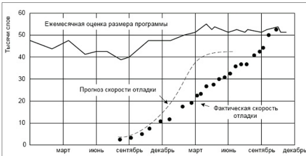
Рис. 8.4 Предсказанная и фактическая скорость отладки
