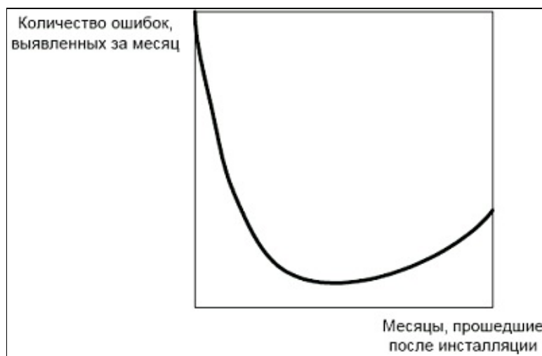
Рис. 11.2 Частота обнаружения ошибок как функция возраста версии программы
