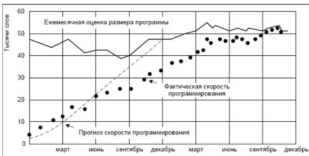
Рис. 8.3 Предсказанная и фактическая скорость программирования Ежемесячная оценка размера программы
